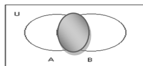
Diagram Venn untuk A \cap B
